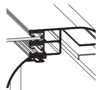
Eficiente sistema de vedação da tampa de vidro
